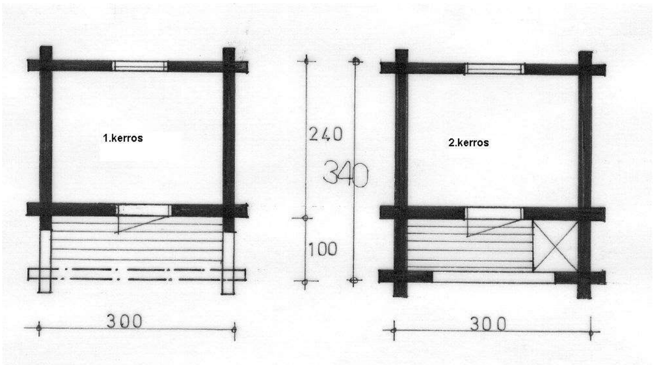
LUHTIAITTA 2 KERROKSENEN
